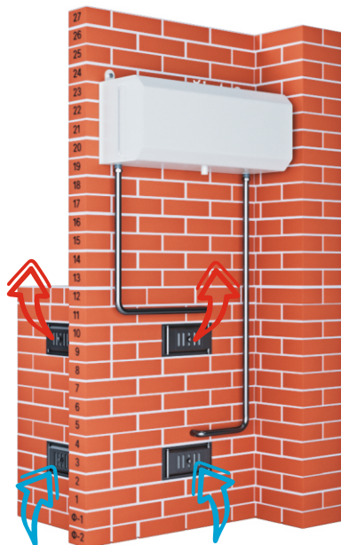
Рис. 8 Пример установки печи в защитном кожухе из кирпича с функцией обогрева комнаты отдыха и моечного отделения
