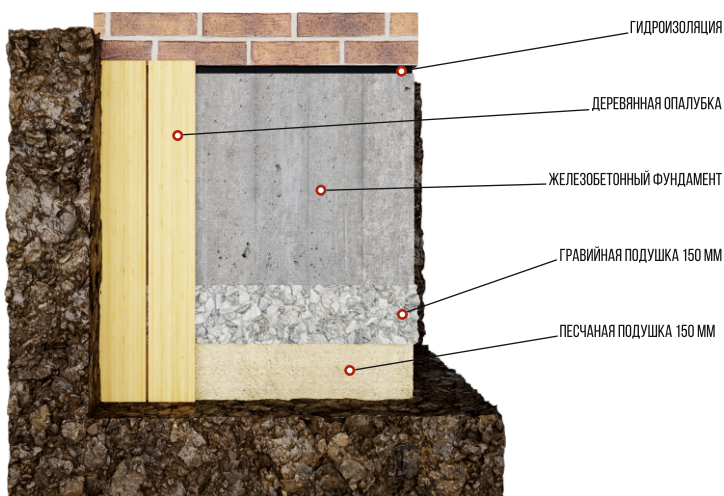
Рис. 13 Схема устройства фундамента
