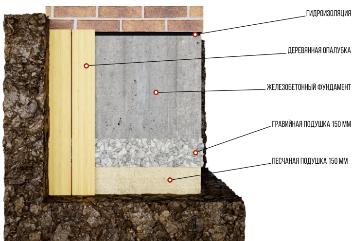
Рис. 9 Схема устройства фундамента
